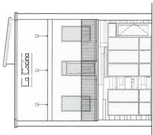
1 New Front Elevation SCALE: 1/8" = 1'-0"
